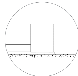
Assemblage de plancher 4 1/4 po x 4 1/4 po FJSPW (T ou U)
