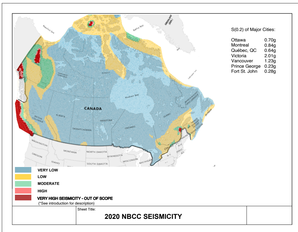
Carte de sismicité au Canada.
