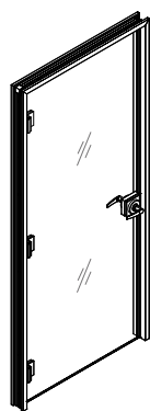
Porte à charnières pour panneaux intercalaires
