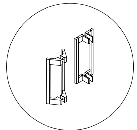
Panneau intercalaire, poignée de porte linéaire (FJHLP)
