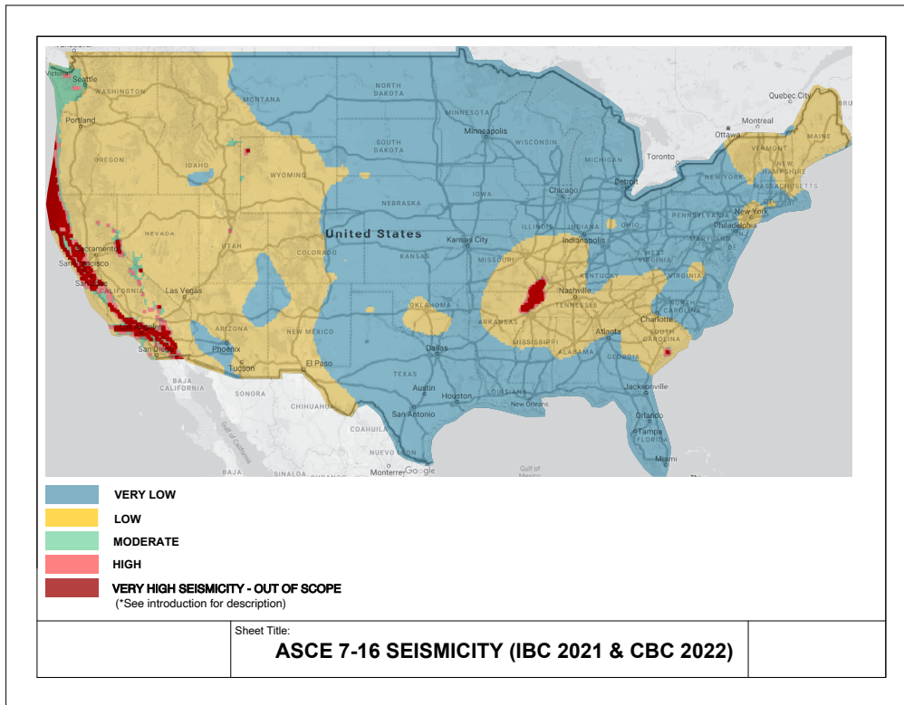
Carte de sismicité aux États-Unis.
