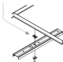
Agrafe de plafond – section inférieure
