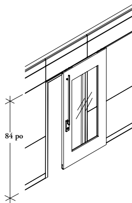
Sectionnelle avec imposte en placage (Landscape illustrée)
