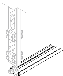
Rail de plancher modulaire (FPKB)
