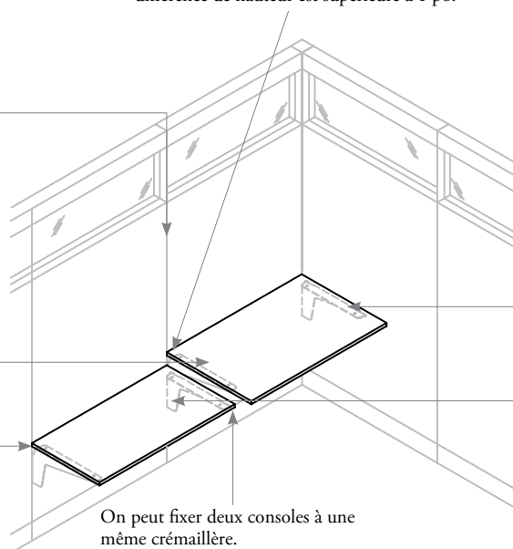
Console sur module
