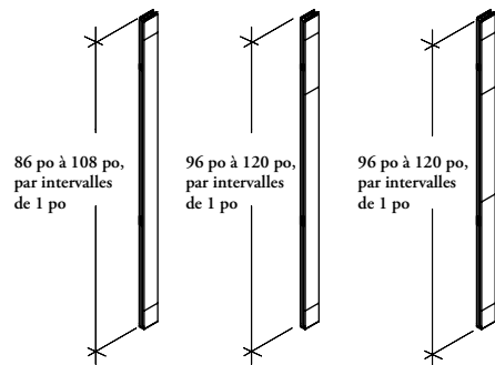
Cloison pleine hauteur
