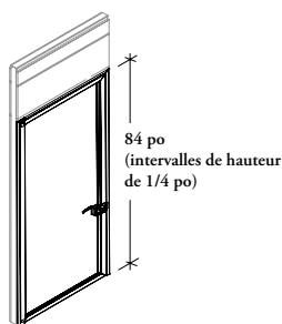
Sectionnelle avec imposte en placage
