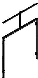
FD S GSJ Ensemble de jambage pour porte coulissante simple en verre
