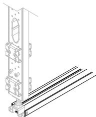
F P K H Ensemble de traverses Xpress
