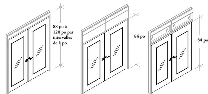
Pleine hauteur
