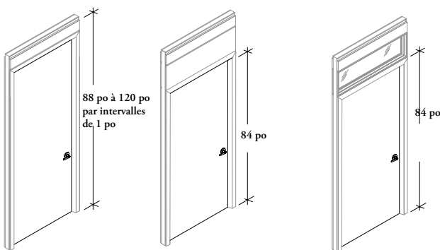
Pleine hauteur Sectionnelle avec imposte en placage Sectionnelle avec imposte vitrée
