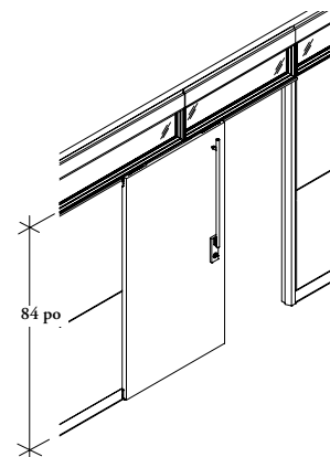
Sectionnelle avec imposte vitrée (Landscape illustrée)
