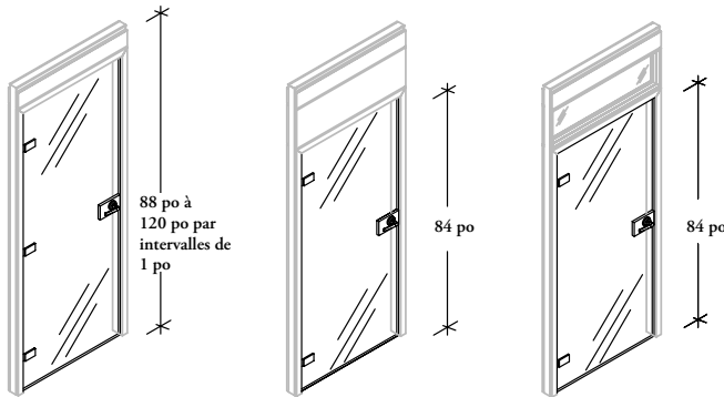
Pleine hauteur Sectionnelle avec imposte en placage Sectionnelle avec imposte vitrée
