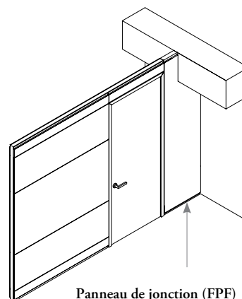
Panneau de jonction (FPF)
