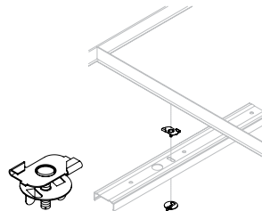
F K V Ensemble de montant Xpress
