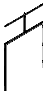
FD DSZF Ensemble de jambage pour porte à charnières double en placage
