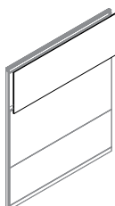
FLRBWM 1 Panneau monolithique recouvert de tissu Landscape – cloison de service (niveau 1 inférieur)
